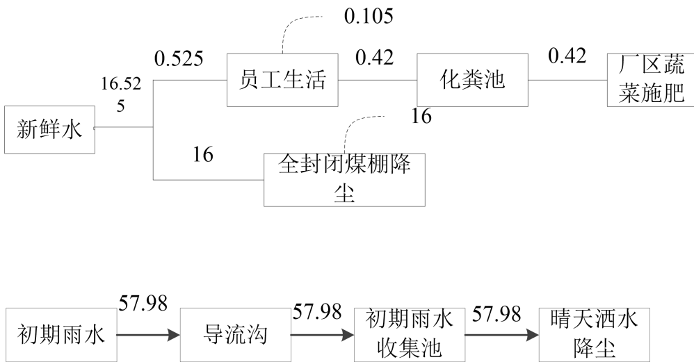
图 2-2 水平衡图（雨天） 单位：m 3 /d
