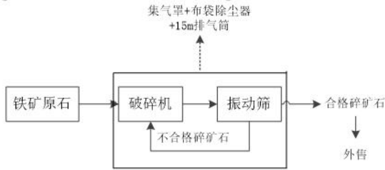
附图 2-6 铁矿破碎筛分产污及工艺流程图
