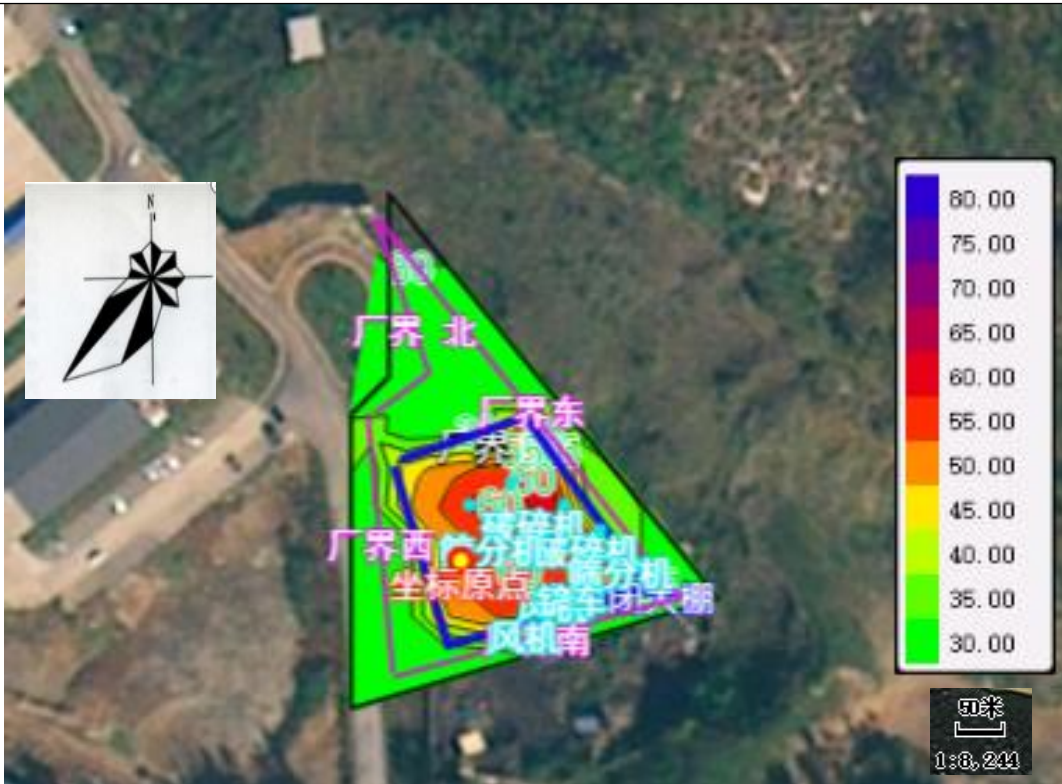
图4-1项目噪声源分布及等声值线图（昼间）
