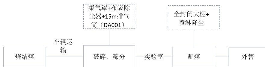
附图 2-4 烧结煤破碎筛分产污及工艺流程图
