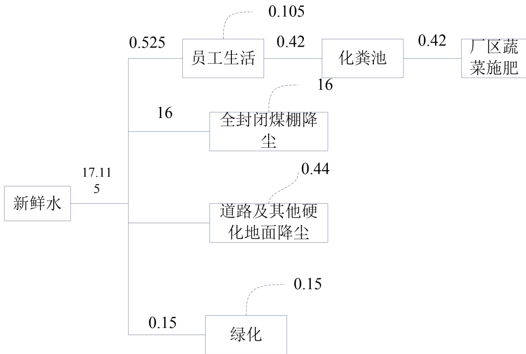
图 2-1 水平衡图（晴天） 单位：m 3 /d
